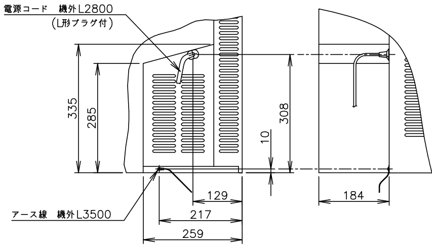
A矢视图 (1/10)
